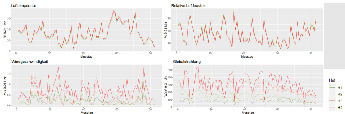
Abb. 7.2: Tagesmittelwerte mikroklimatischer Messwerte zwischen 9.00 und 21.00 Uhr basierend auf den Messwerten in den vier Innenhöfen in Potsdam-Drewitz.
