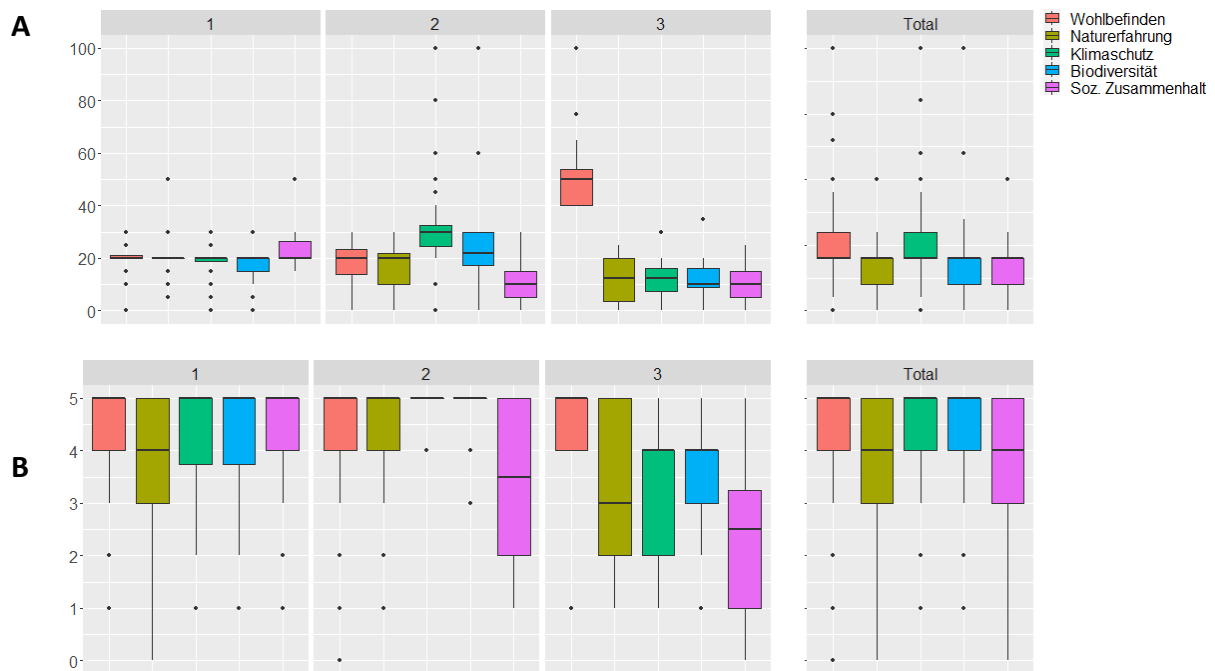
Abb. 7.4 Gewichtung der Ökosystemleistungen: A) Median, 25%- und 75%-Quantile der Gewichtung mit insgesamt 100 Punkten über alle Ökosystemleistungen für die drei Cluster und die gesamte Stichprobe („Total“); B) Median, 25%- und 75%-Quantile der Bewertung von Ökosystemleistungen von 1 („sehr unwichtig“) bis 5 („sehr wichtig“) für die drei Cluster und die gesamte Stichprobe („Total“).
