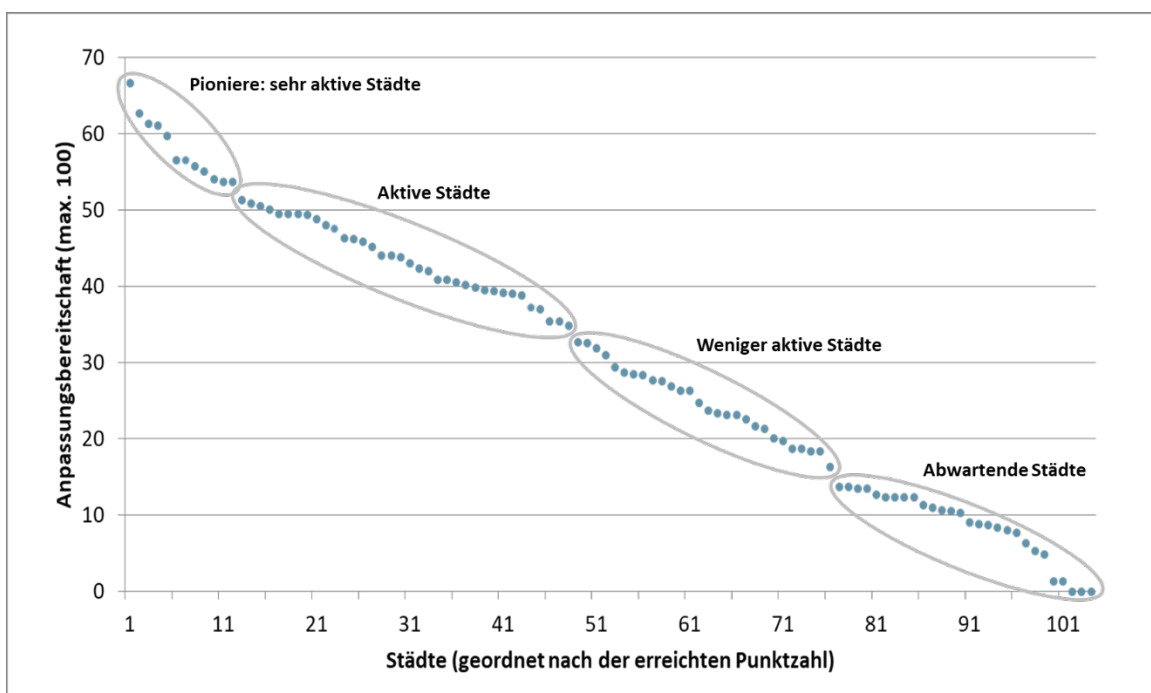
Abb. 2.4: Verteilung der 104 Städte entsprechend ihrer erreichten Punktzahl für ‚adaptation readiness‘ (vgl. Otto et al. 2021b).
