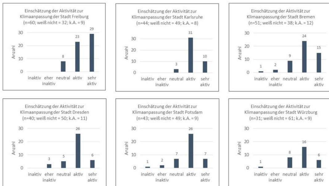
Abb. 2.5: Darstellung der sechs Städte mit der besten Fremdrezeption (von zwölf Städten).
