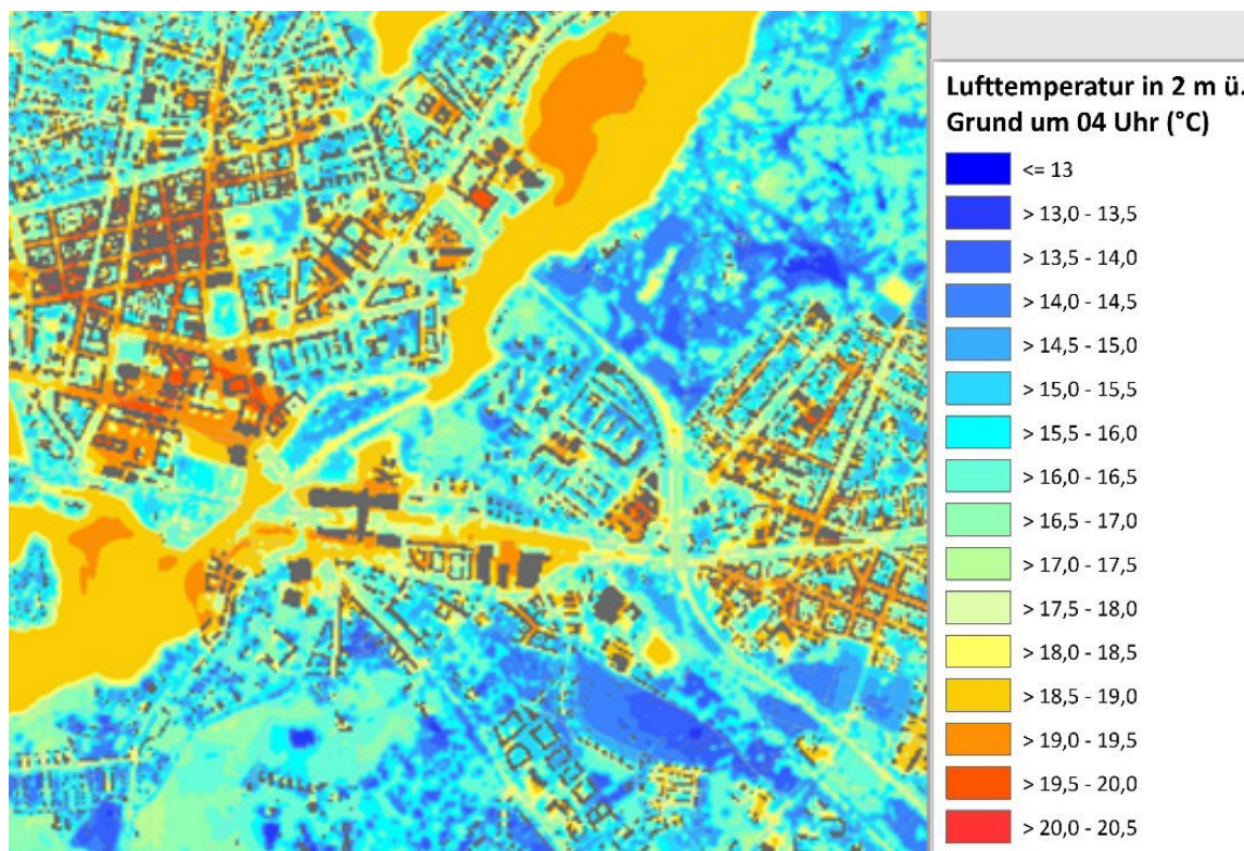
Abb. 5.1: Temperaturfeld im Bereich der Potsdamer Innenstadt zum Zeitpunkt 4 Uhr morgens (2m über Grund).
