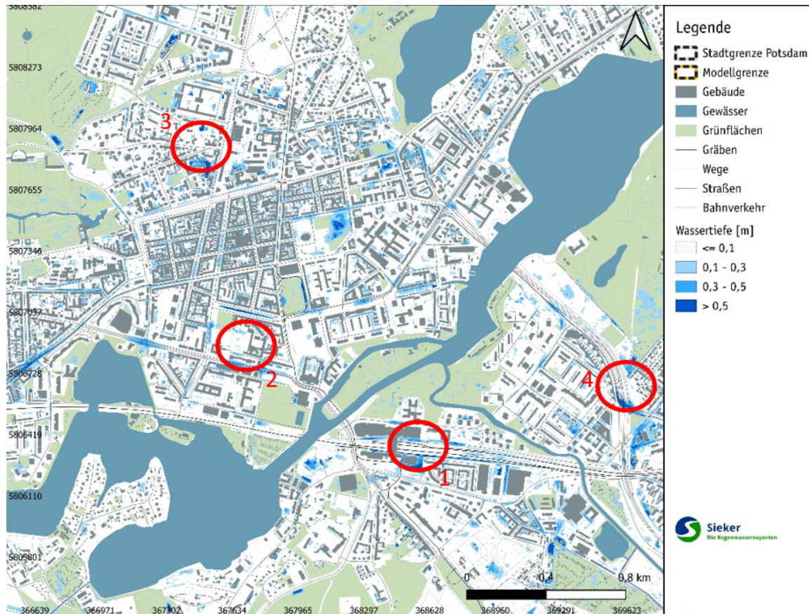
Abb. 5.7: Ergebnisse der 2D-Oberflächenmodellierung für den Bereich der Potsdamer Innenstadt.
